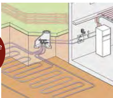
Variante 1: Flächenkollektoren
